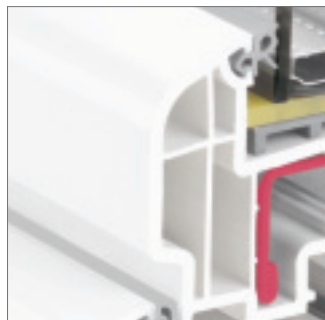
Designflügel abgerundet
