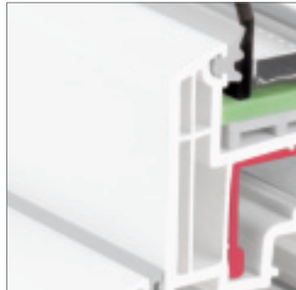
Designflügel flächenversetzt
